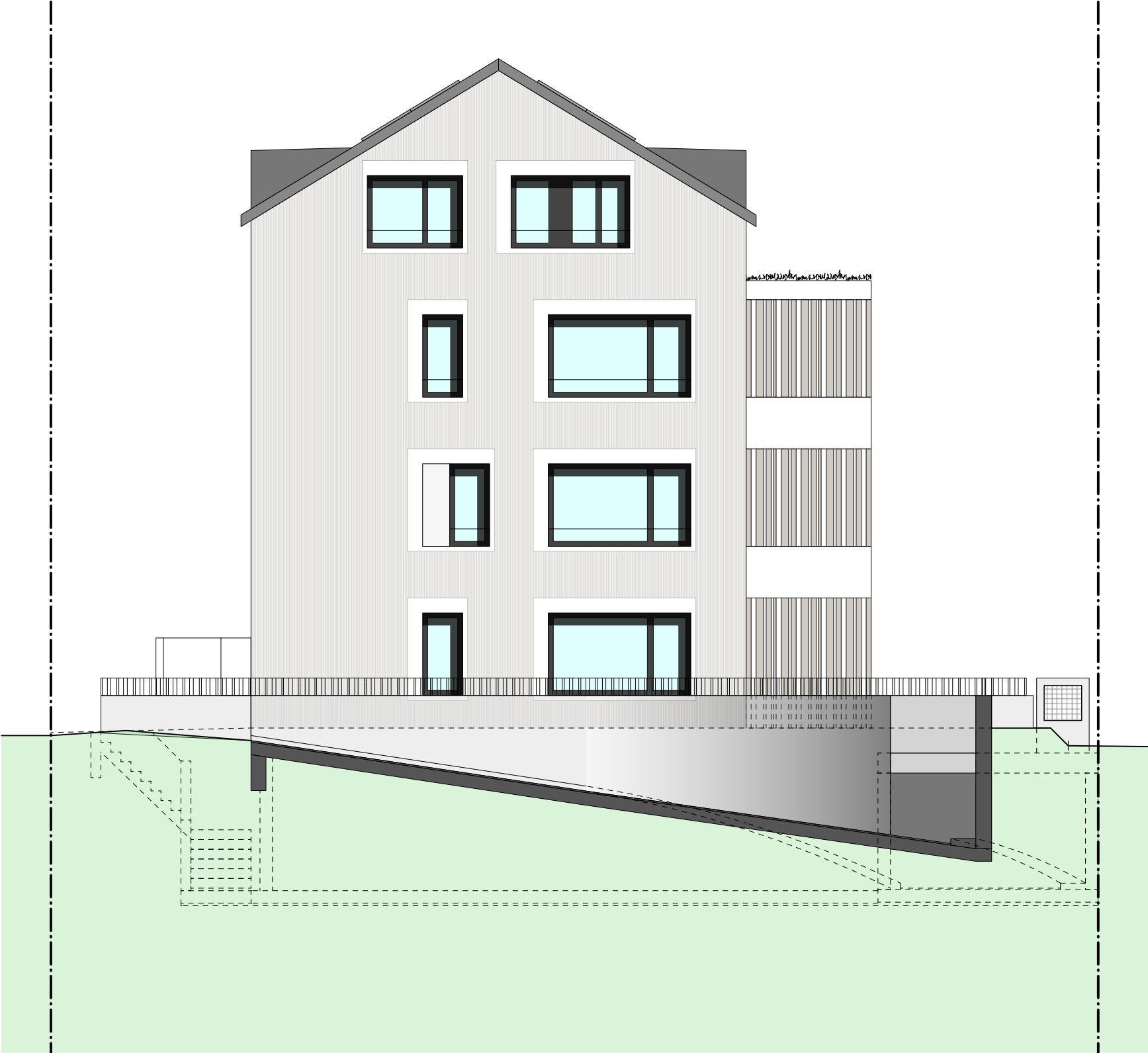
Nordfassade
